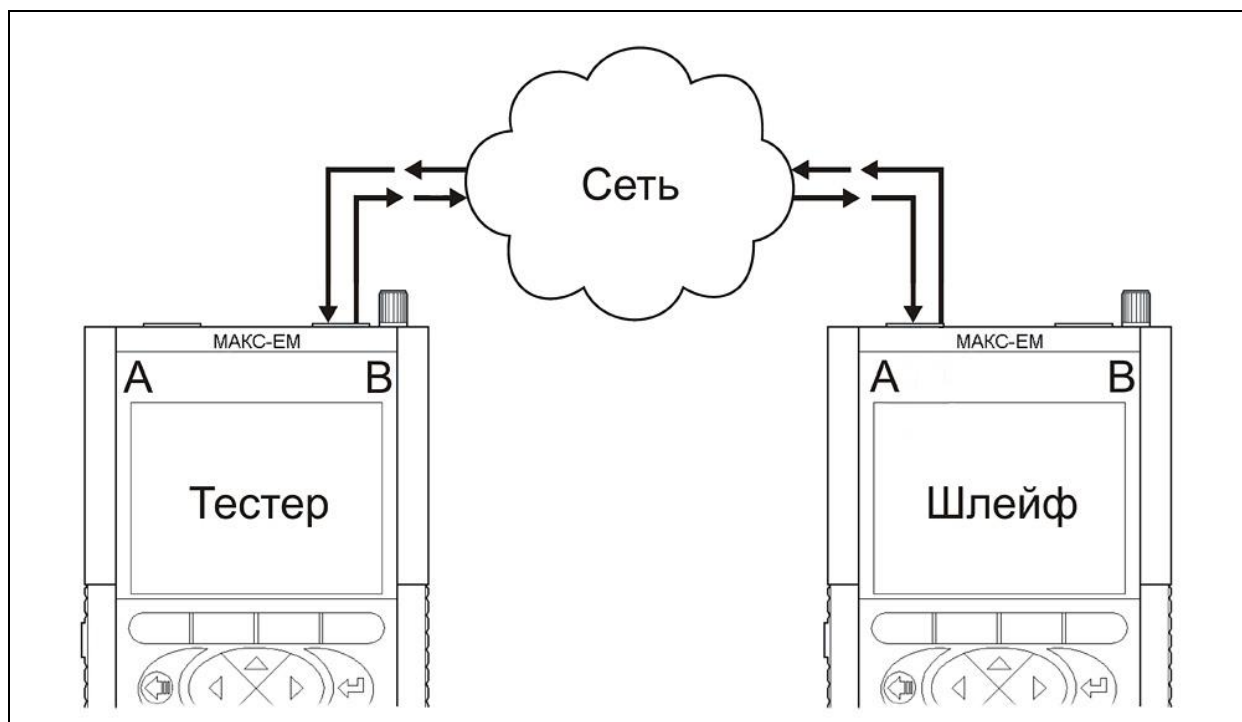
Рисунок 10.7 - Схема «С» подключения прибора в режиме тестирования асимметричных каналов
