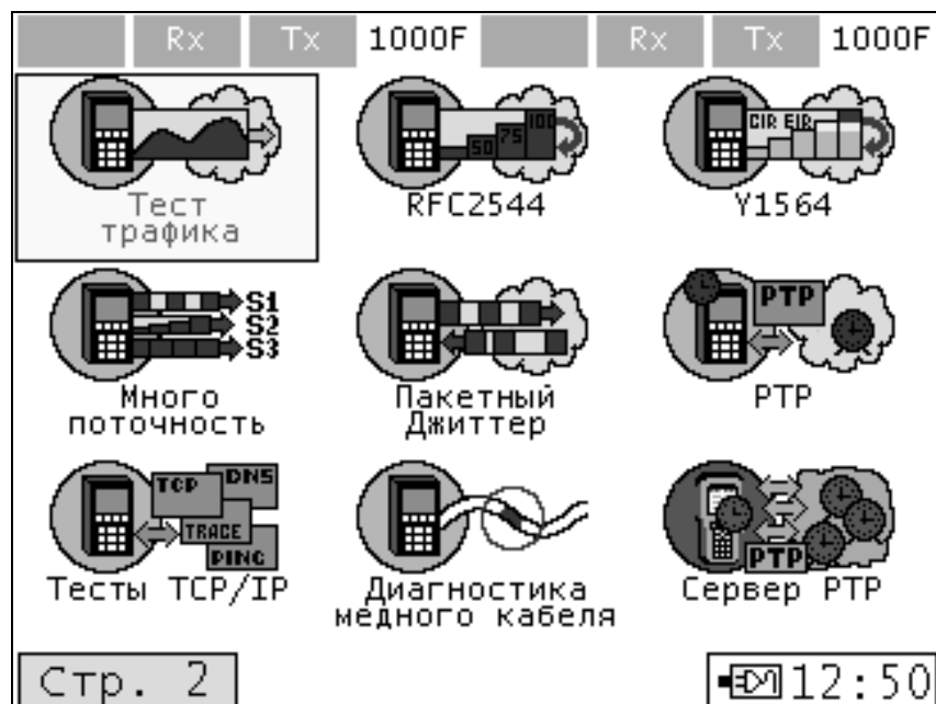
Рисунок 10.2 - Первая страница меню «Измерения»
