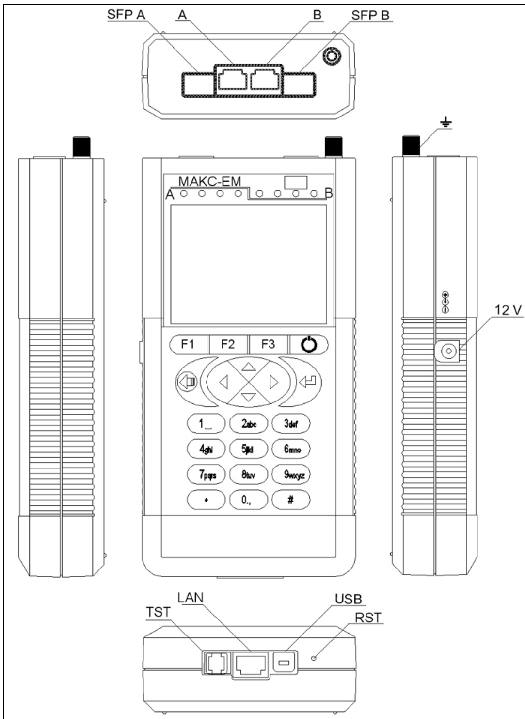
Рисунок 4.2 - Схема расположения разъемов прибора
