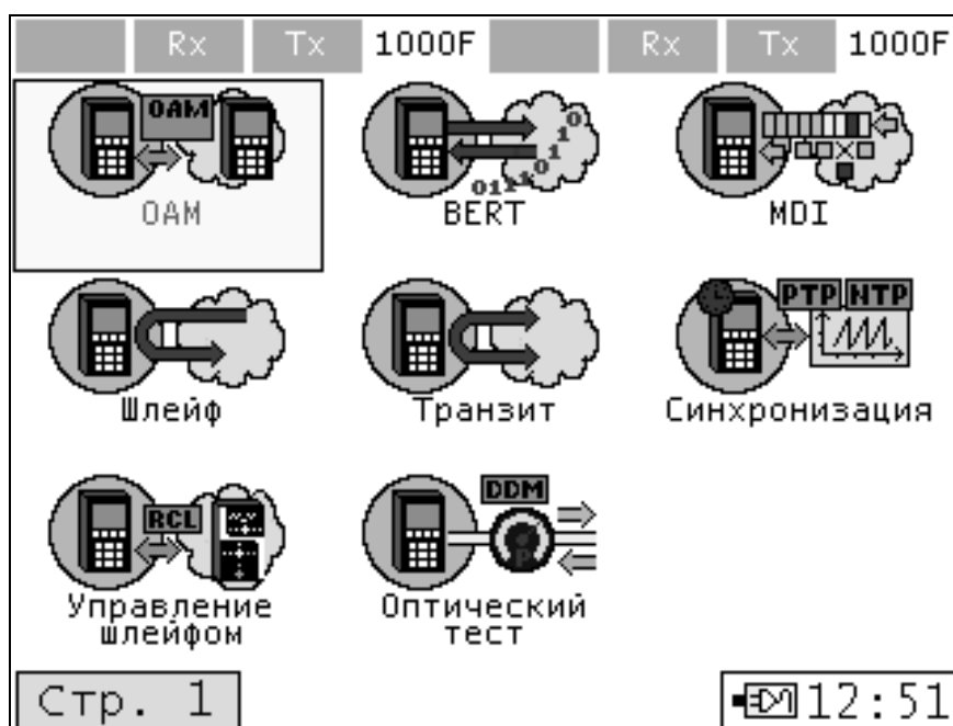
Рисунок 10.3 - Вторая страница меню «Измерения»
