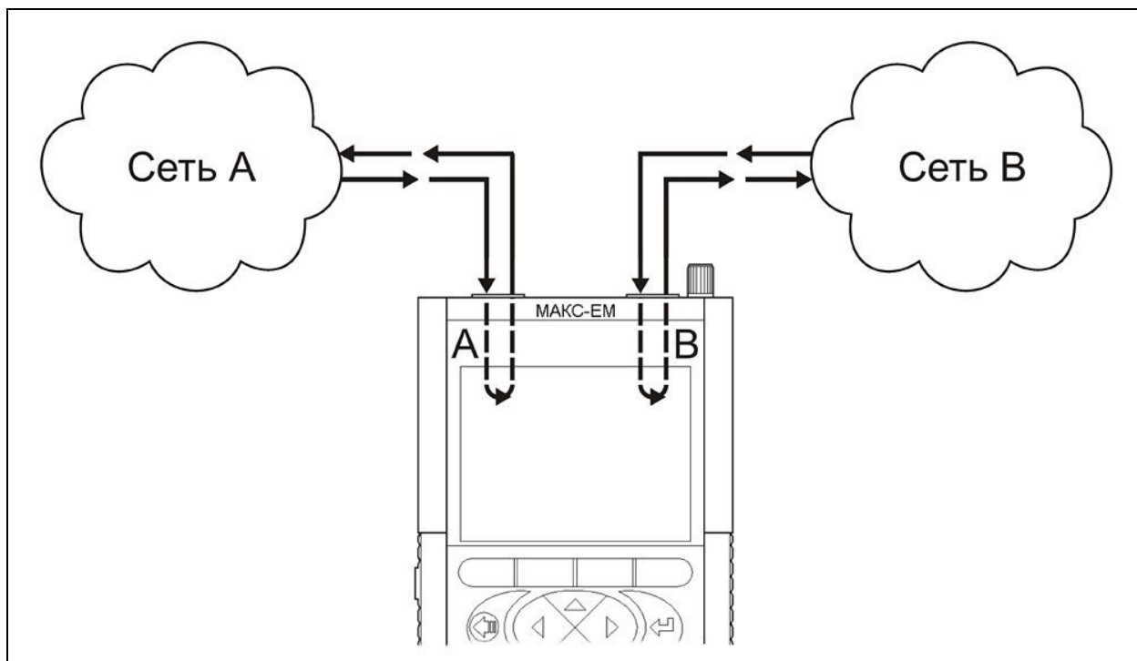
Рисунок 10.26 - Схема подключения в режиме Шлейф
