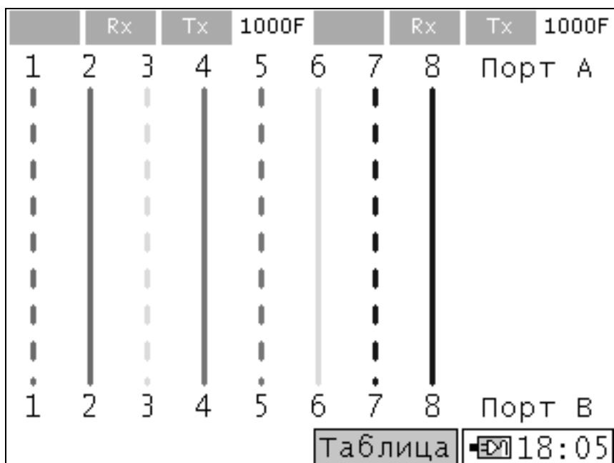
Рисунок 10.21 - Диагностика медного кабеля. Схема коммутации
