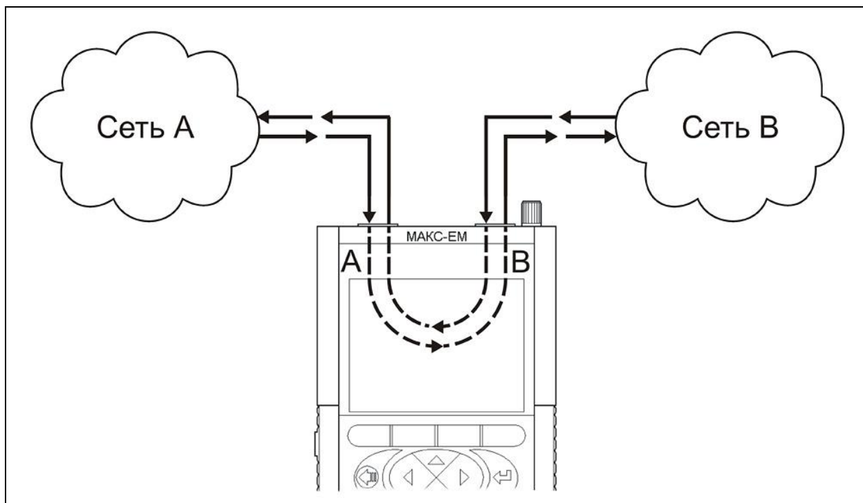
Рисунок 10.27 - Схема подключения в режиме Транзит
