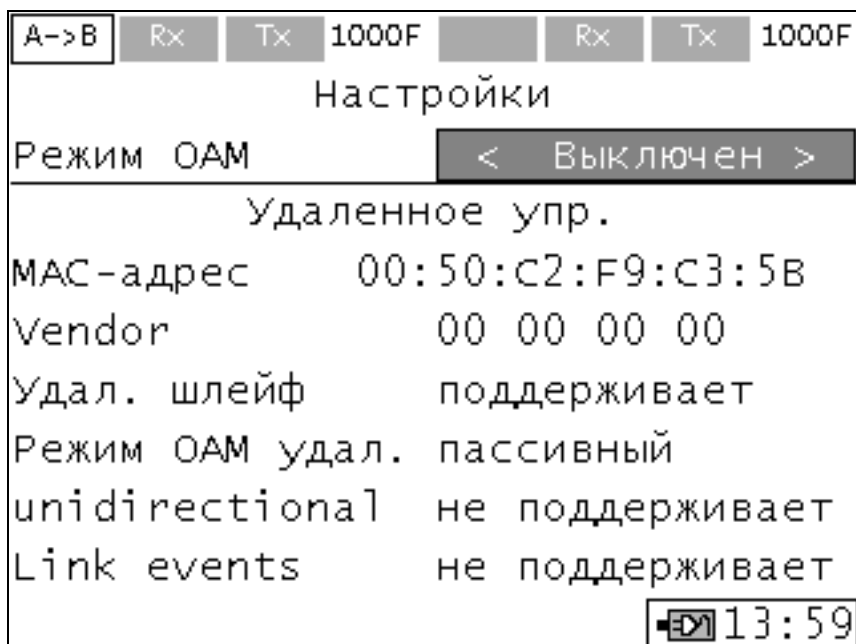
Рисунок 10.23 - Удаленное управление OAM
