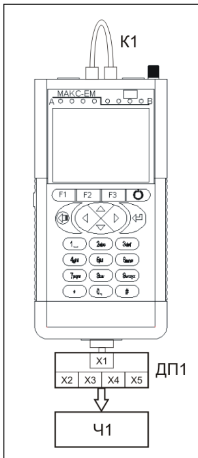
Рисунок 11.7 - Схема подключения при проведении поверки
