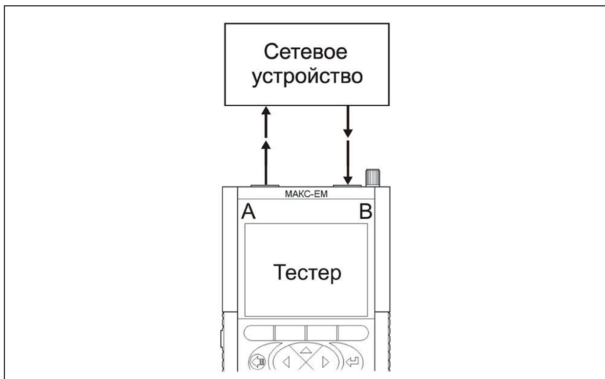
Рисунок 10.6 - Схема «В» подключения прибора в режиме однонаправленного тестирования
