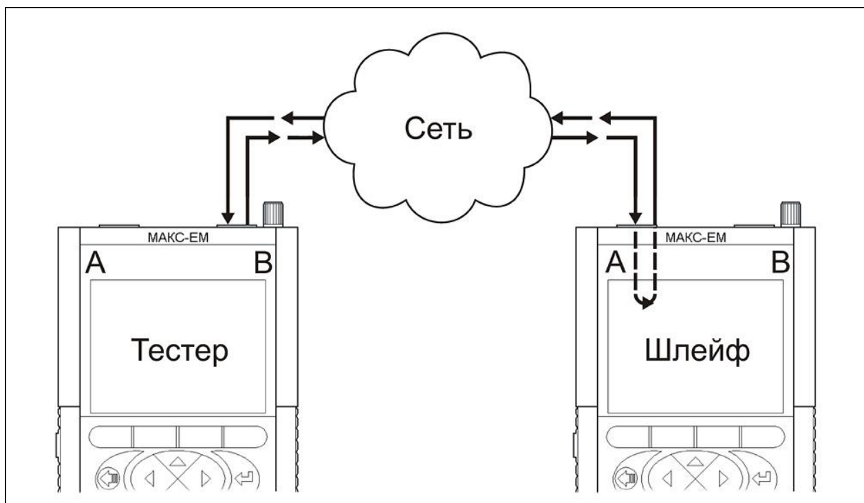
Рисунок 10.5 - Схема «А» подключения прибора в режиме тестирования симметричных каналов
